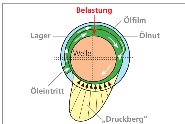
Bild 2: Druckverteilung in einem Gleitlager
